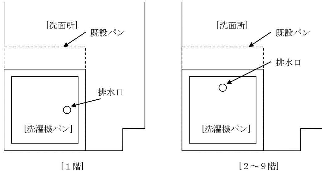
図 14 64×64cm の洗濯機パンの設置（奇数号室の配置を例として表示）
