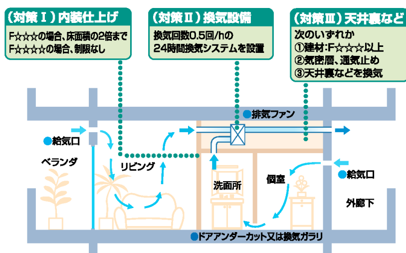
図1 共同住宅の場合のシックハウス対策（国土交通省）
