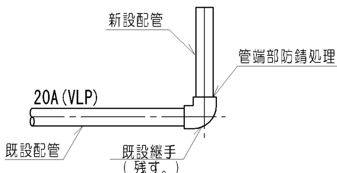
図3 新しい配管の接続
