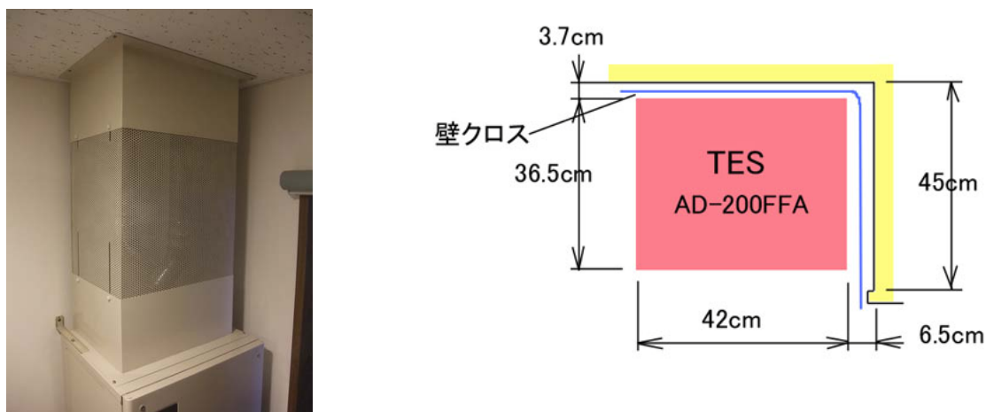
図 53 TES の背面のクロス貼り
