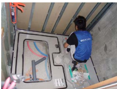
新しいユニットバスの床 部材の組立て状況
