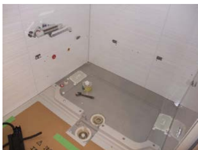
浴槽下の排水用パンを取り付けた状態
